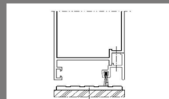
provedení bez prahu (lišta 3 mm + kartáč)
