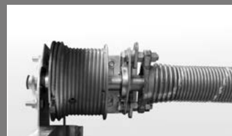
torzní pružina vyvažuje hmotnost vrat
