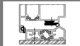
hliníkový podlahový práh s PTM (20 mm)
