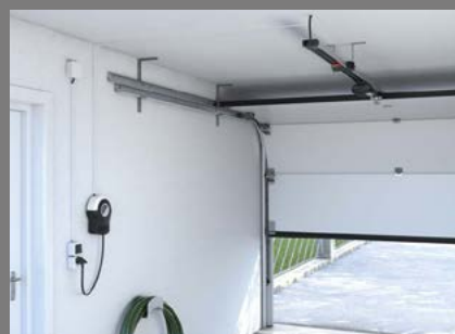
Řídicí jednotka v prostoru garáže
