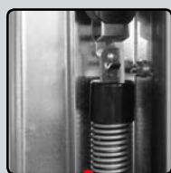
Tažná pružina vyvažuje hmotnost vrat
